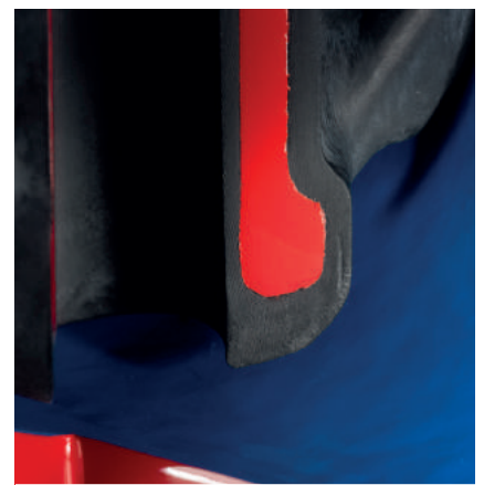
Quando la valvola viene riaperta, la gomma riprende la sua forma originale
