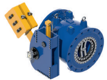
Attuatore oleodinamico con contrappeso
