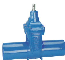
Serie 32/40 Saracinesca con innesto lungo per tubi in ghisa DN80-300 PN16 Ghisa sferoidale
